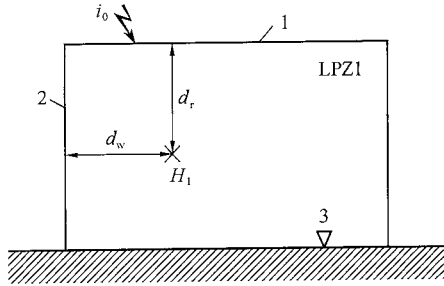
图 D. 2. 1 闪电直接击于屋顶接闪器时 LPZ1 区内的磁场强度 1—屋顶；2—墙；3—地面
