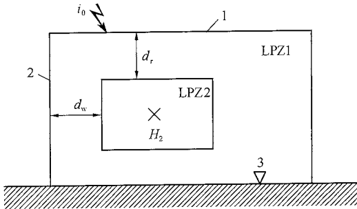
图 D. 2. 2 LPZ2 等后续防护区内部任意点的磁场强度的估算 1—屋顶；2—墙；3—地面
