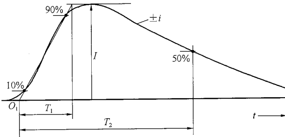
图 C.0.1-2 短时雷击波形参数
