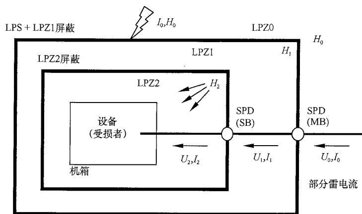
(a) 采用空间屏蔽和“协调配合的 SPD 防护”的 LPMS ——对于传导浪涌 ( U_2 < U_0 和 I_2 < I_0 ) 和辐射磁场 ( H_2 < H_0 )，设备得到良好的防护
