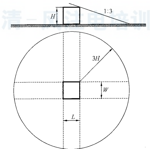
图 B. 5. 3-1 孤立建筑物的截收面积 A_d
