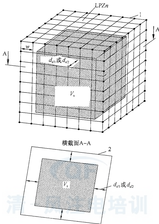
图 5.3.2 LPZn 内用于安装电子信息系统空间 1—屏蔽网格；2—屏蔽体； V_s —安装电子信息系统空间； d_{s/1} 、 d_{s/2} —空间 V_s 与 LPZn 的屏蔽体间应保持的安全距离； w —空间屏蔽网格宽度
