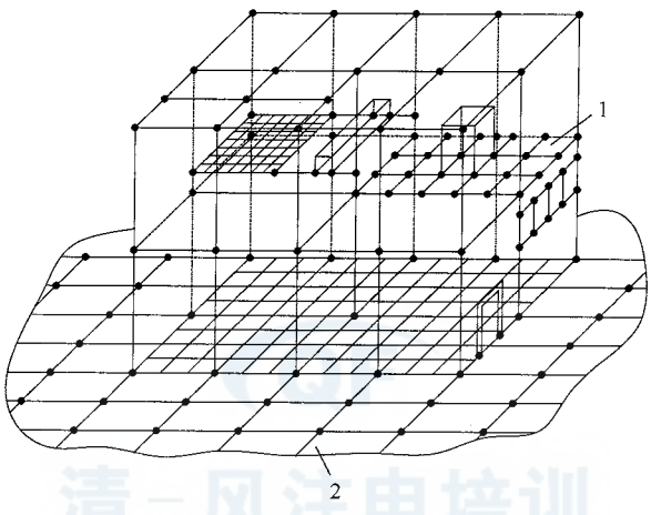
图 5.2.3 由等电位连接网络与接地装置组合构成的三维接地系统示例 1—等电位连接网络；2—接地装置
