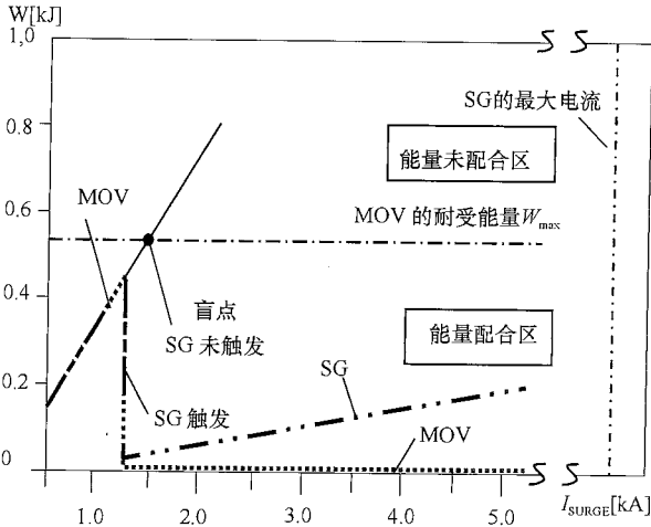
图 14 SG 和 MOV 的能量配合原理
