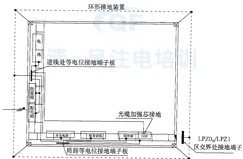
图 15 移动通信基地的接地
