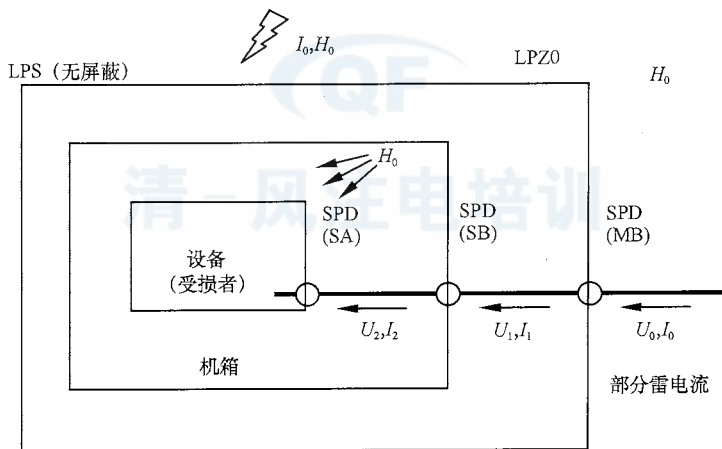
(d) 仅采用“协调配合的 SPD 防护”的 LPMS ——对于传导浪涌 ( U_2 \ll U_0 和 I_2 \ll I_0 ), 设备得到防护; 但对于辐射磁场 ( H_0 ) 却无防护作用
