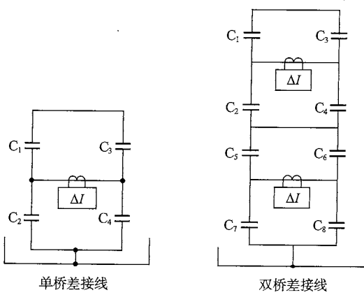
图 6.1.2-3 单星形电容器组桥式差电流保护原理接线
