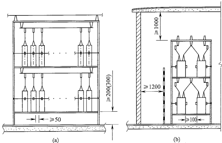
图 1 并联电容器组安装示意图
