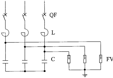
图 4.2.8 相对地避雷器接线
