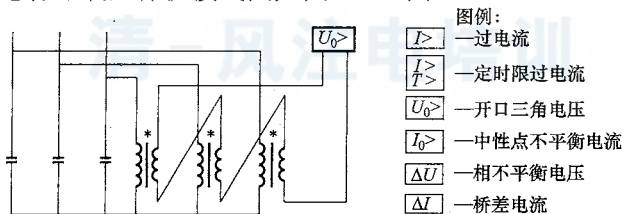
图 A.5 开口三角电压保护接线
