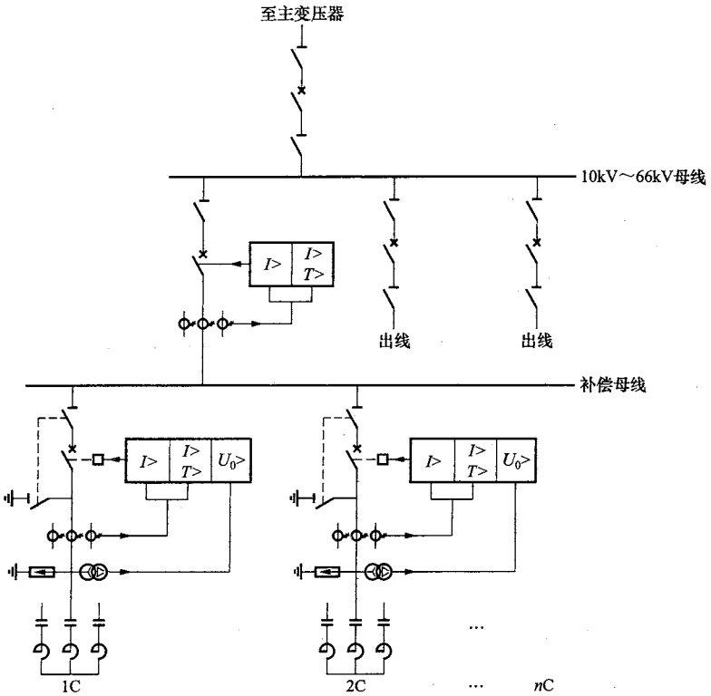
图 A.8 多路电容器组采用专用补偿母线的分级保护设置
