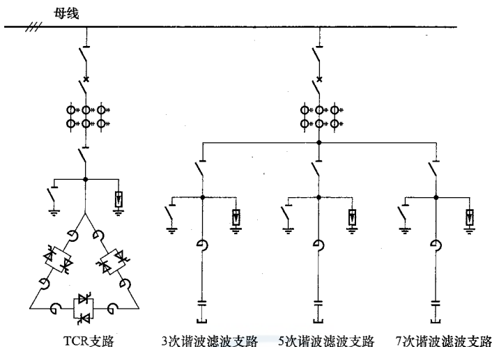
图 A.4 TCR+FC 接线方式
