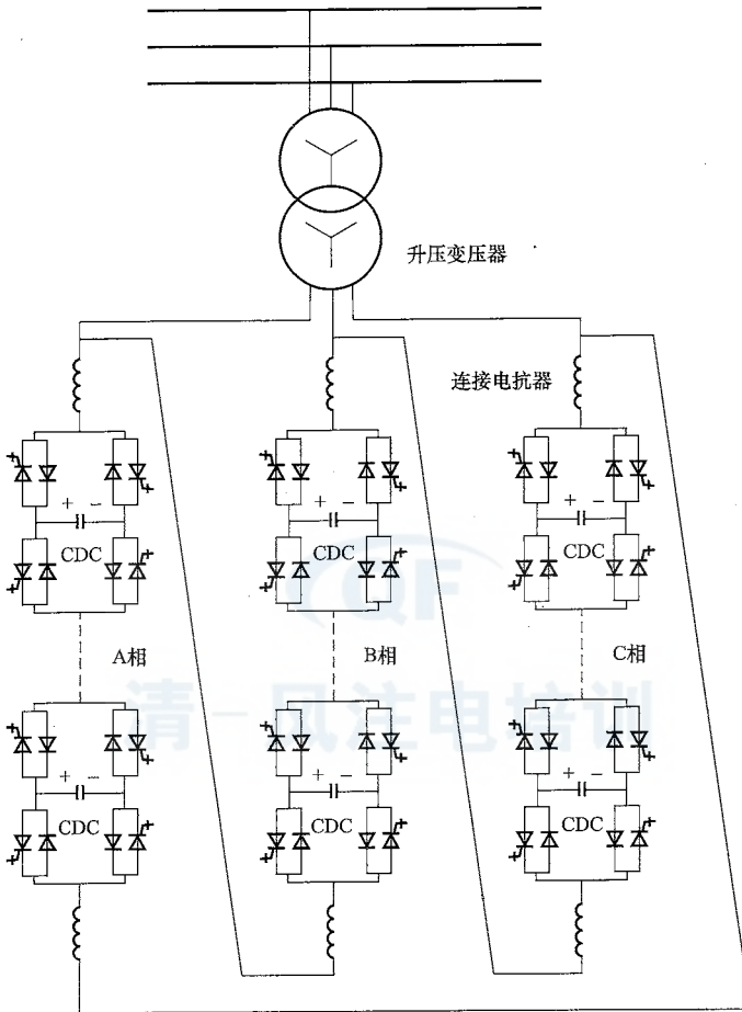
图3 链式 STATCOM 接线
