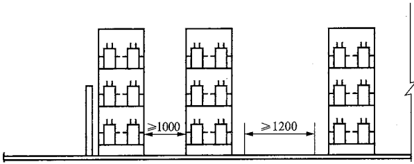
图6 户外电容器组通道设置示意图
