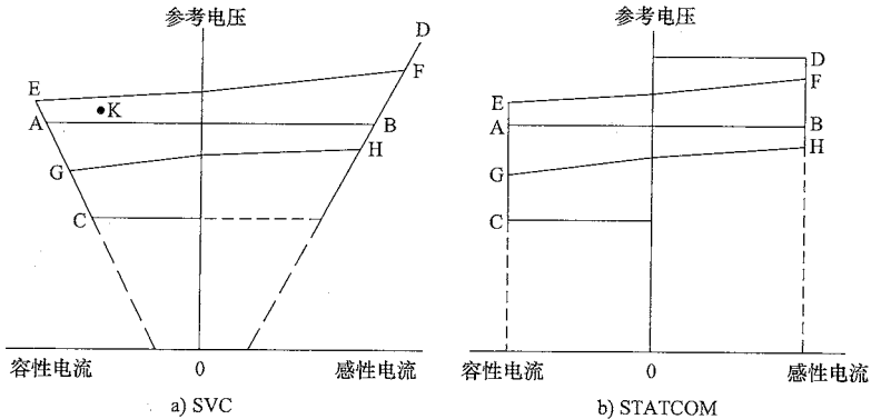
图 4 SVC 及 STATCOM 运行特性
