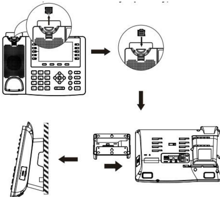
图 2 - 壁挂式安装
