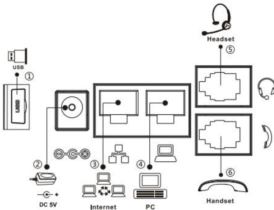
图 3 - 设备连接
